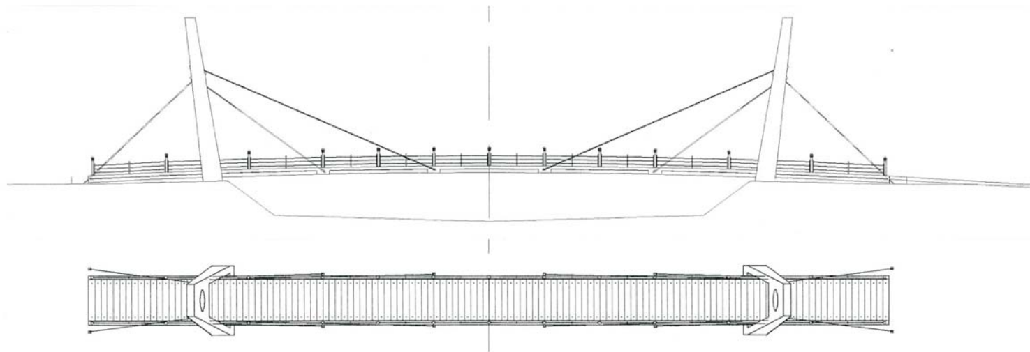
planta i alçat
