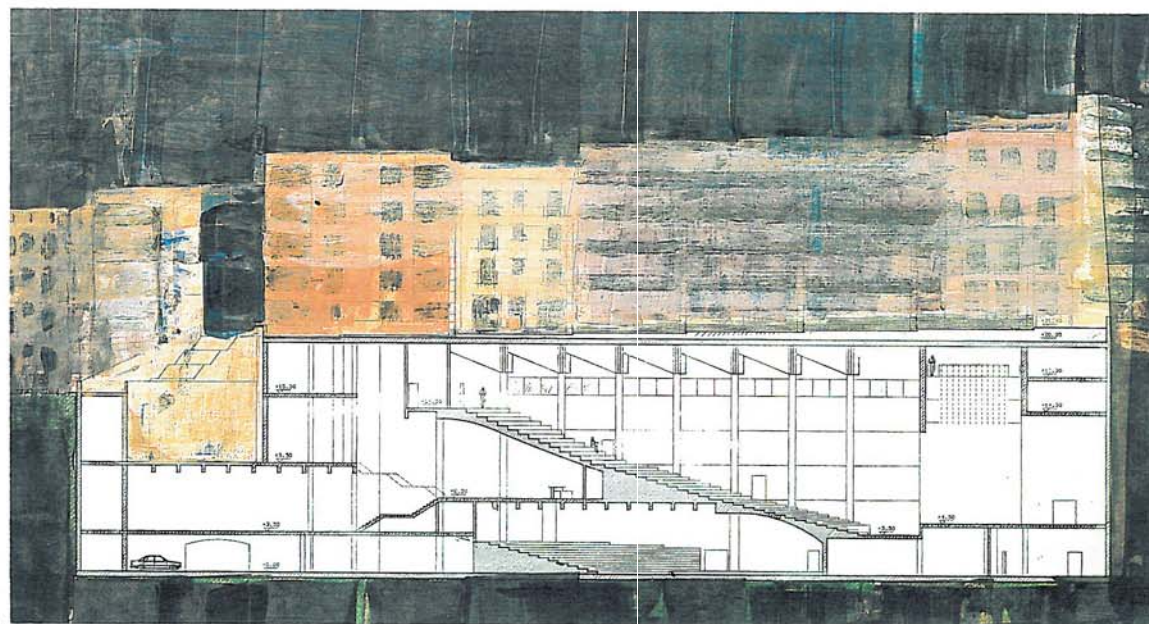
Secció
