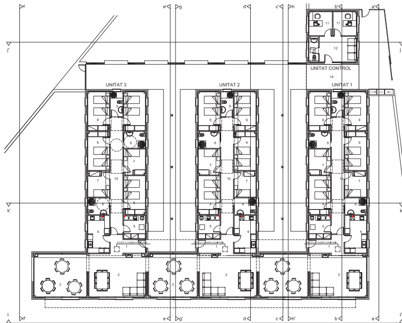
Planta general
